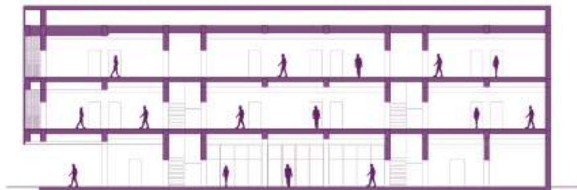
SEZIONE LONGITUDINALE
